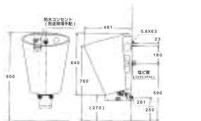
標準取付図 (LS800DMの場合)
