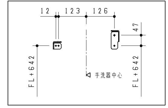
※1 手洗器固定金具ねじ位置詳細(1:10)
