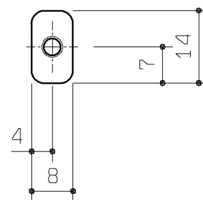
B矢視
