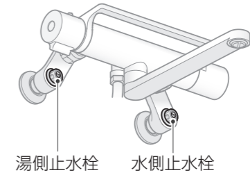
壁付
