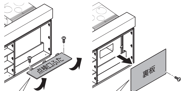
1 点検口ふた
