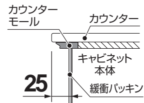
【共通側面図】
