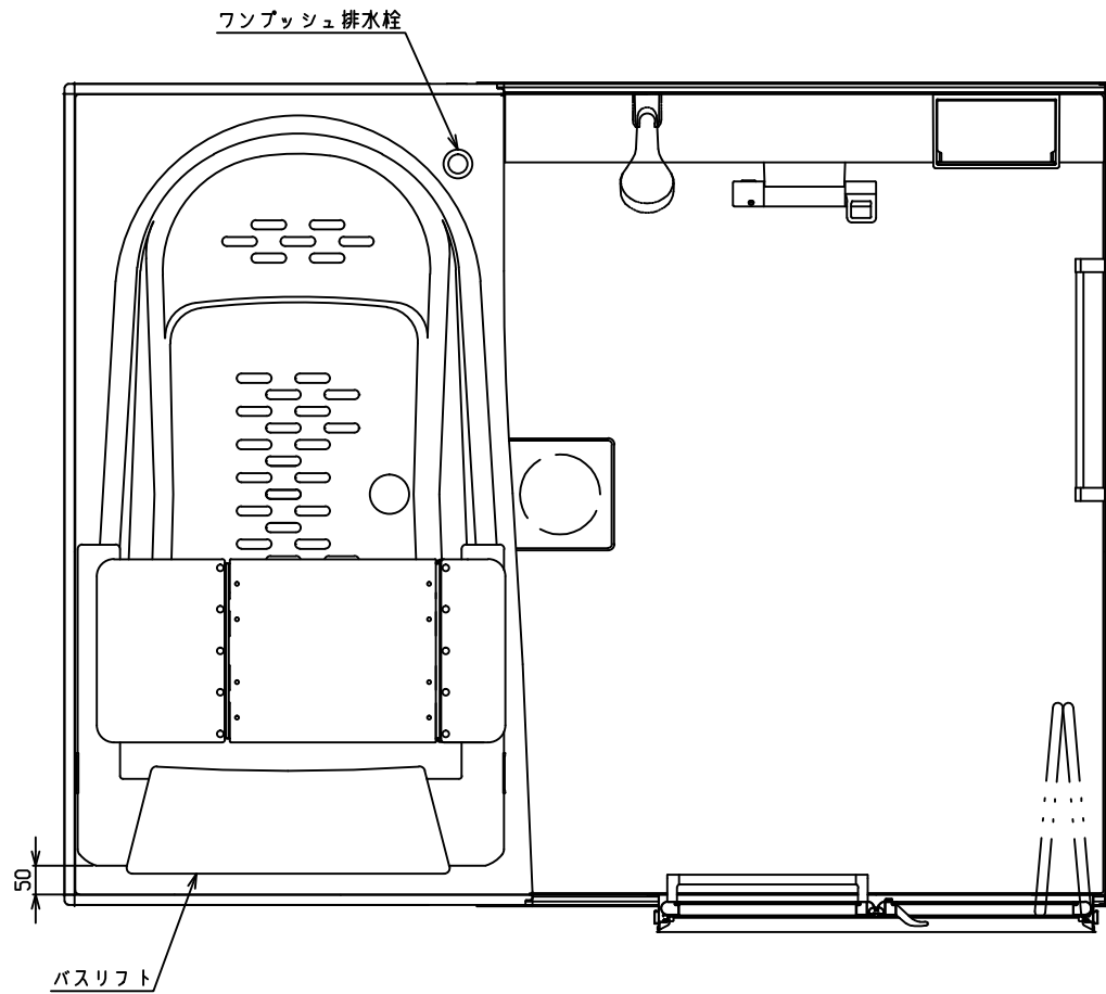
1400ラウンド浴槽
