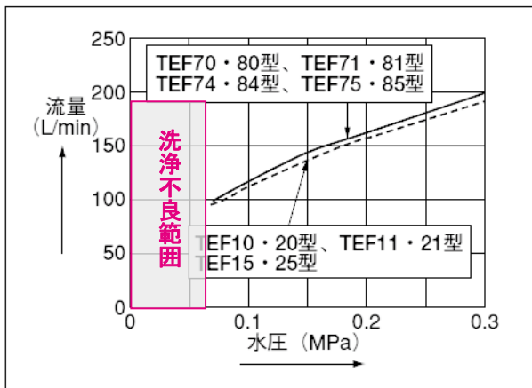
(流量線図)
