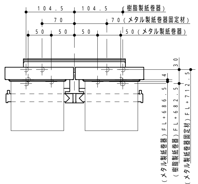
紙卷器固定部詳細
