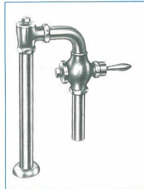
床給水床上排水形 低圧用フラッシュバルブ T 173
