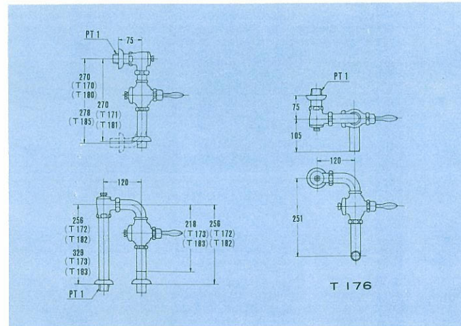
大小便兼用フラッシュバルブ (腰掛便器 C 14用) T 185
