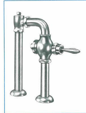
床給水床排水形 大小便兼用フラッシュバルブ T 182
