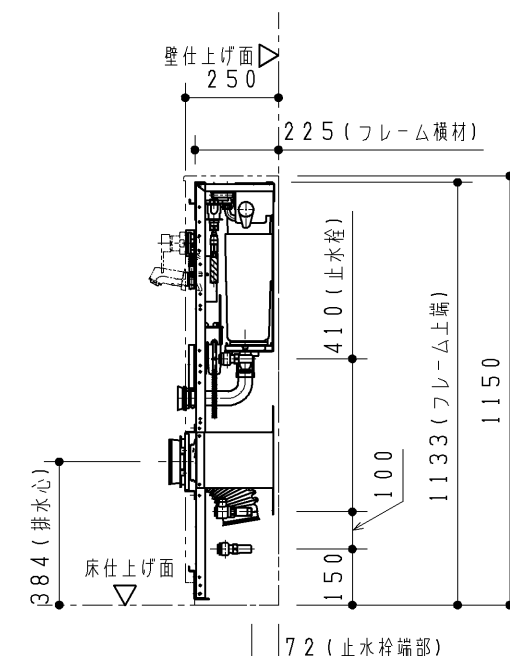
R 視図
