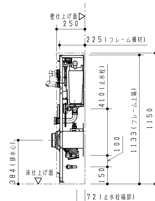
R 視図
