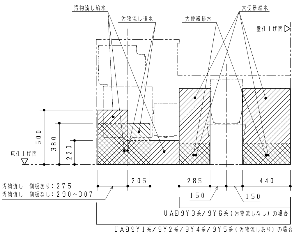
UAD9Y2系・UAD9Y5系 （汚物流し側板なし）の場合
