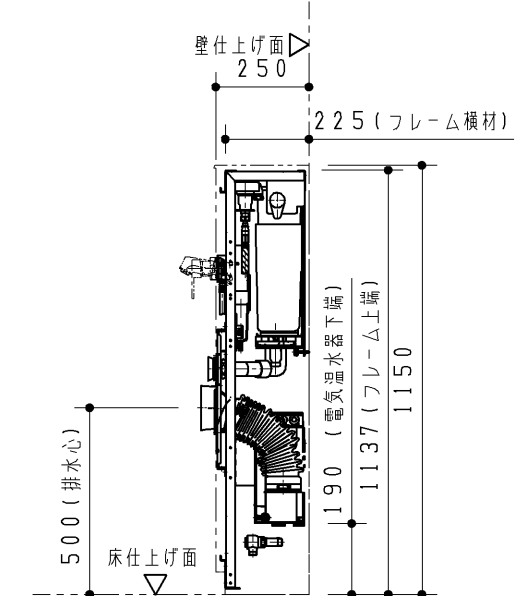
R 視 図
