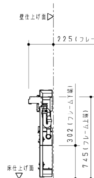
P 視図
