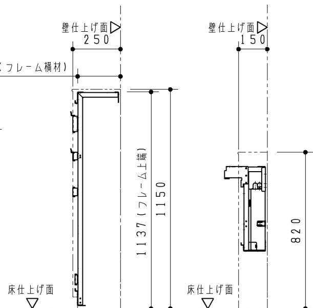
R 視図
