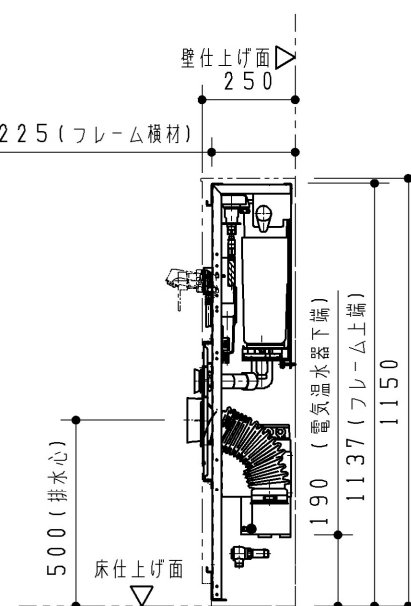
T 視図
