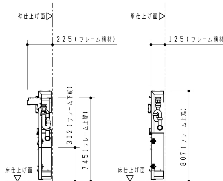
P 視図
