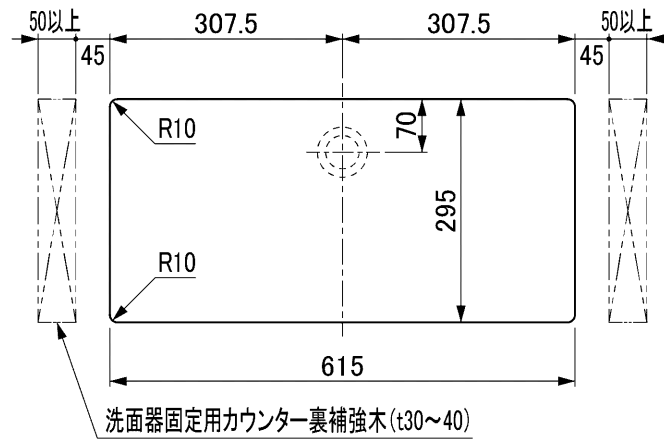
カウンター切込寸法
