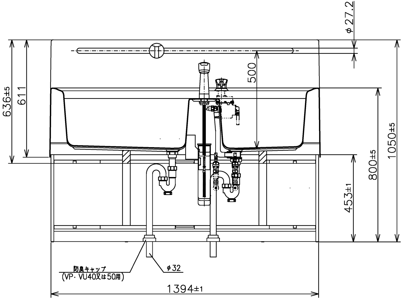
断面A-A
