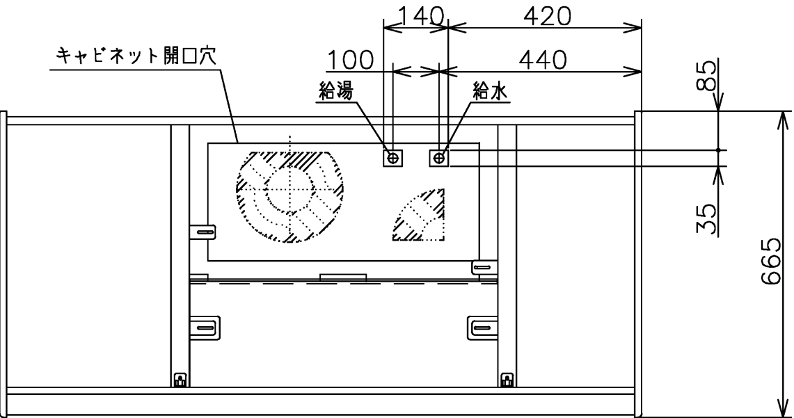
給水・給湯管接続範囲(床取出し)
