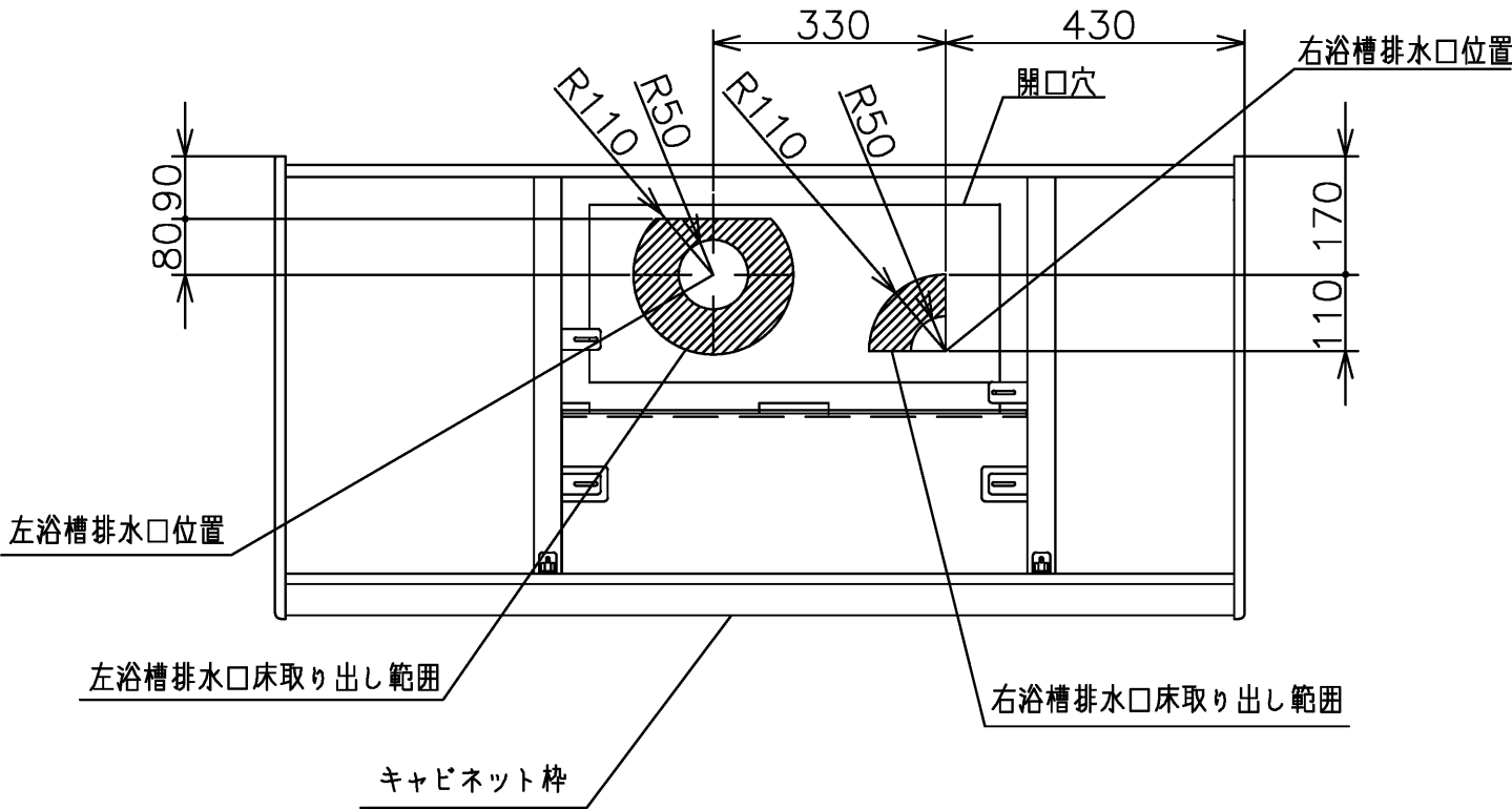
排水管接続範囲
