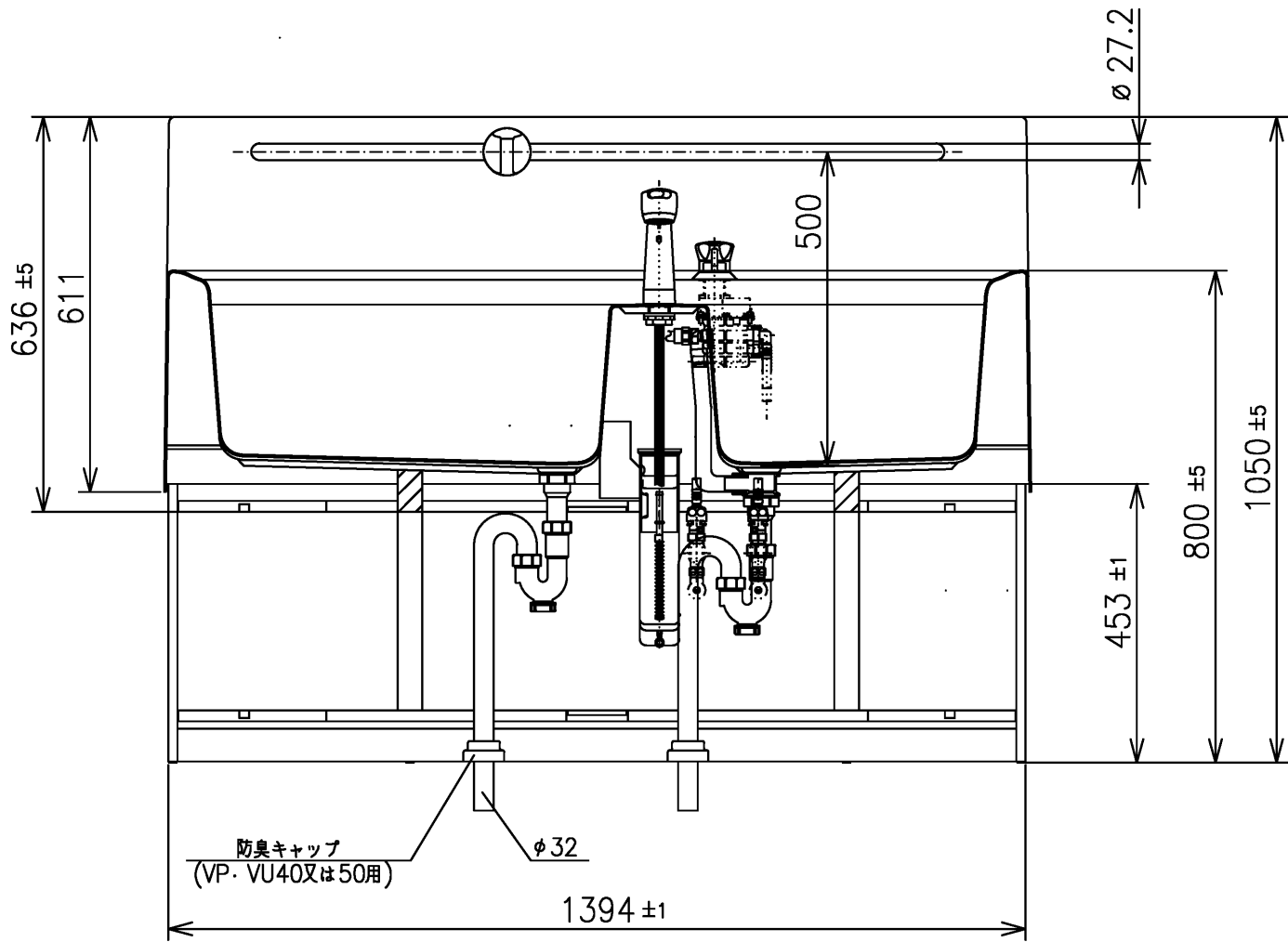
断面A-A
