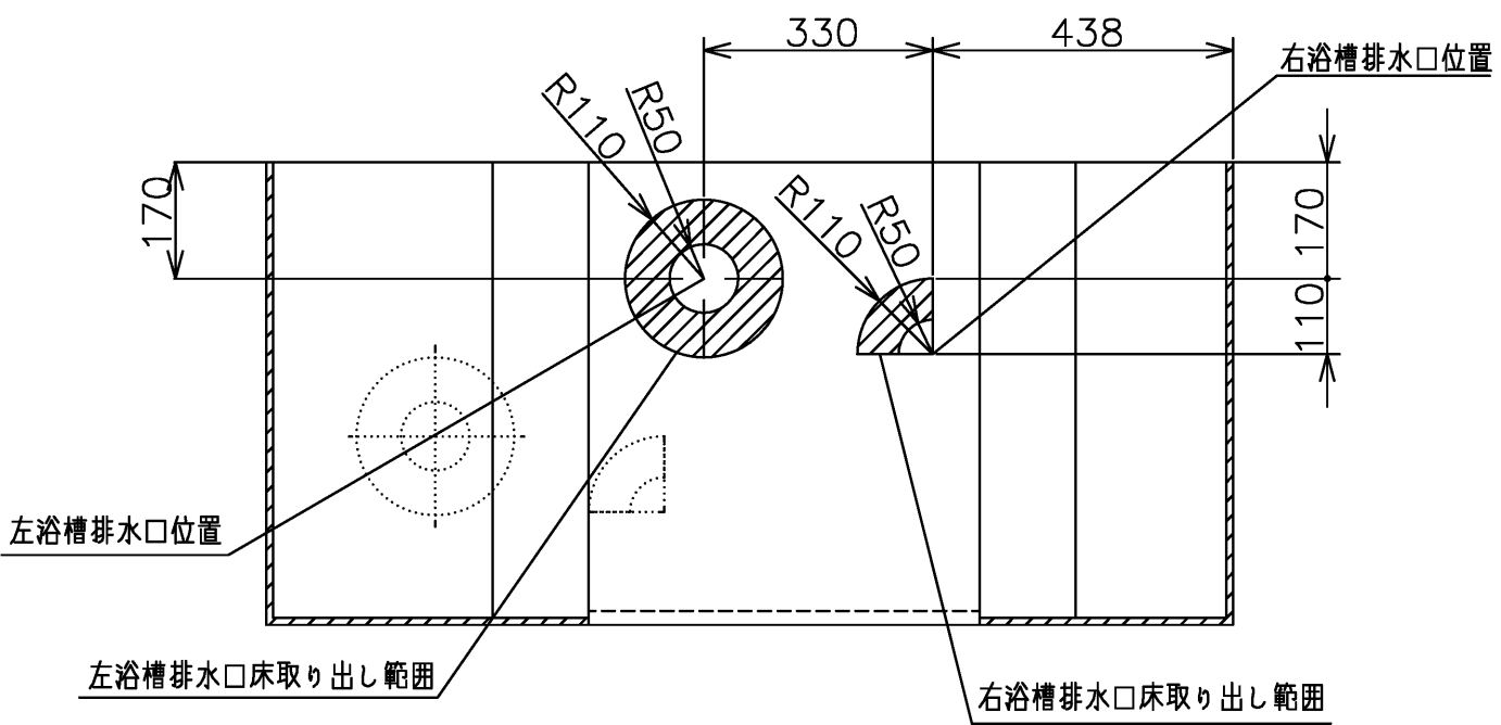
排水管接続範囲
