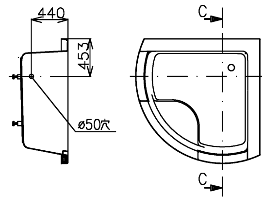
断面C-C
