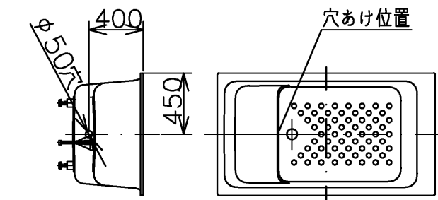
追焚用穴あけ可能位置(1:40)
