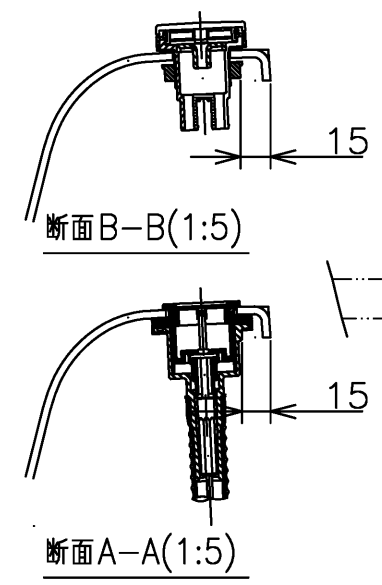
サヤ管固定部詳細図
