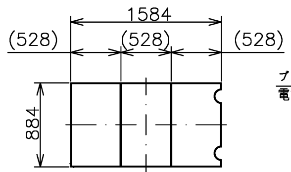
組合せふろふた(1:40)
