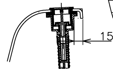
断面A-A(1:5)
