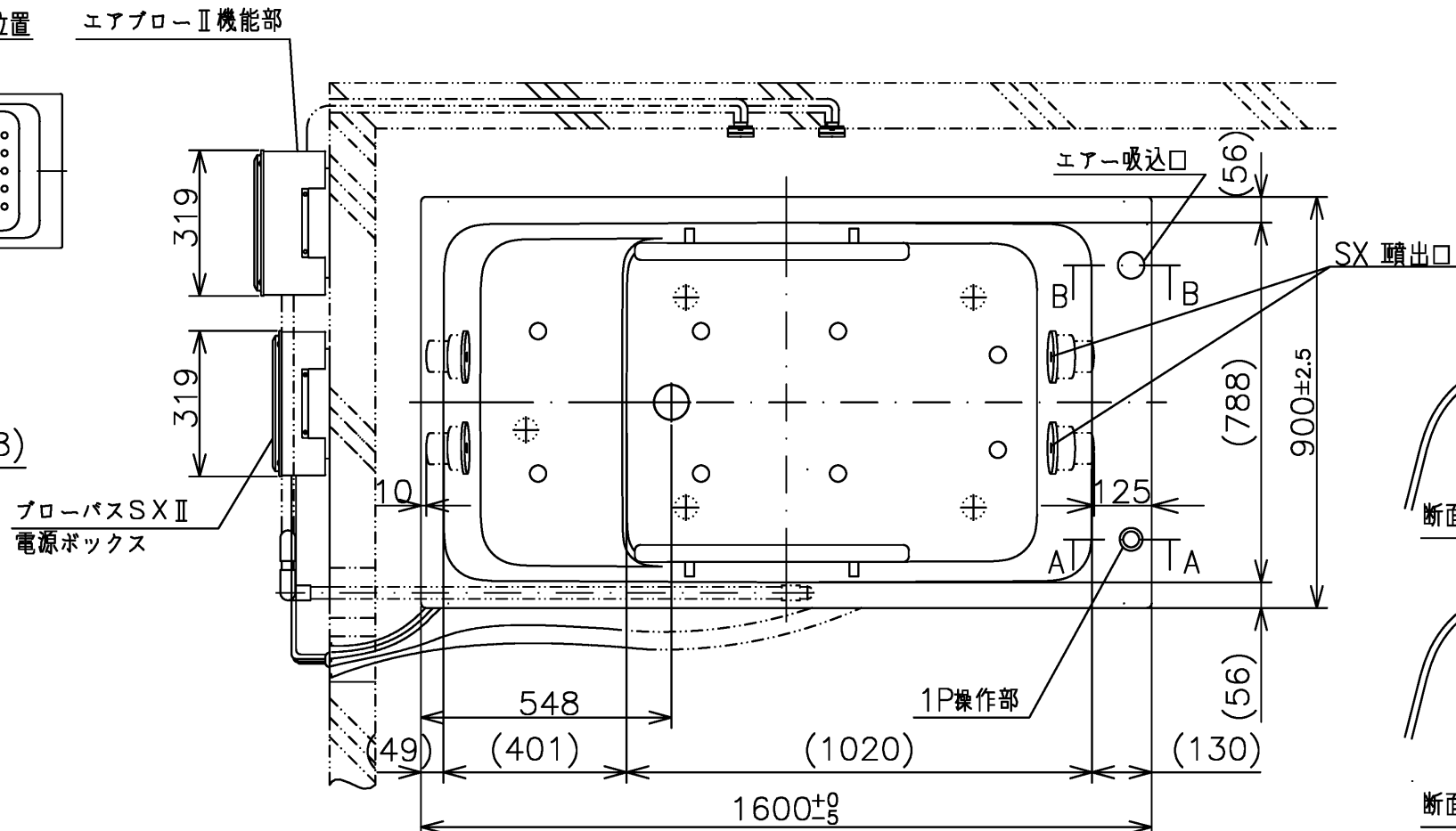
追焚用穴あけ可能位置(1:40)
