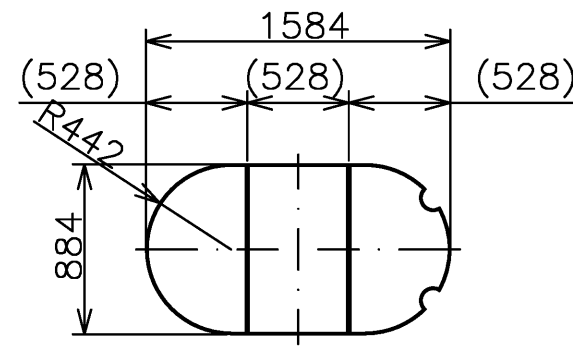
組合せふろふた(1:40)
