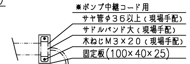
サヤ管固定部詳細図
