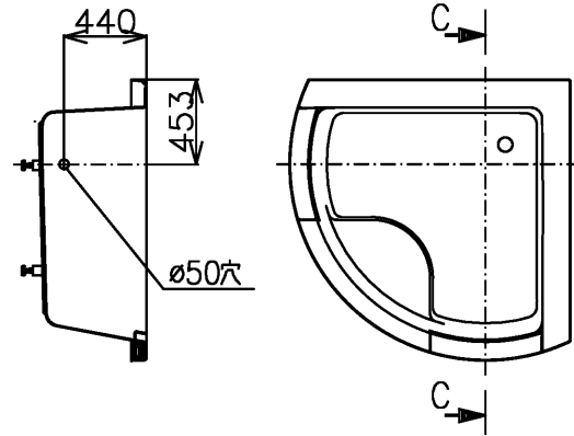
断面C-C
