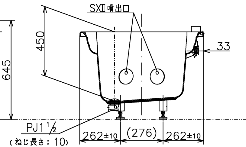
断面A-A
