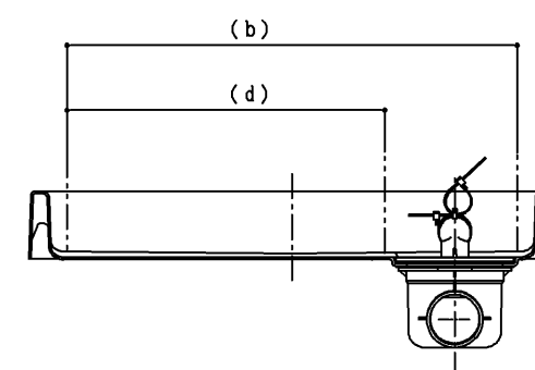
断面B-B
