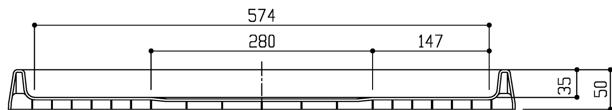
断面B-B
