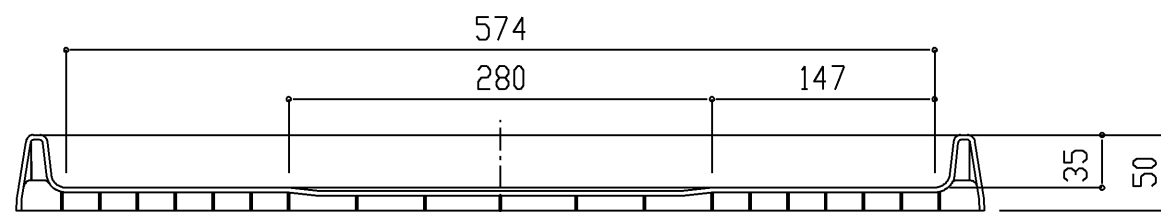
断面B-B
