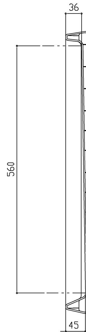
断面A-A
