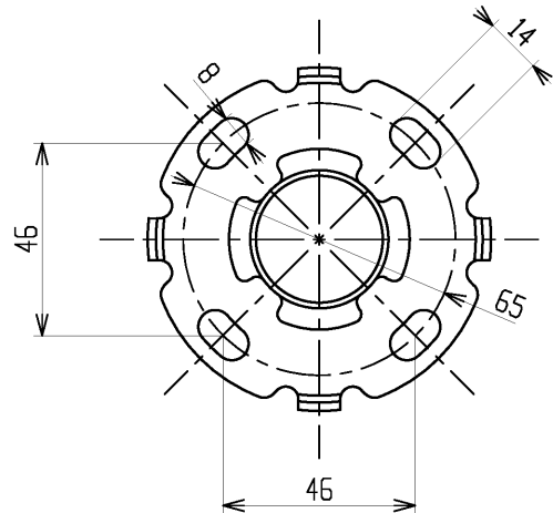
取付座詳細(1:2)
