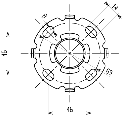
取付座詳細(1:2)
