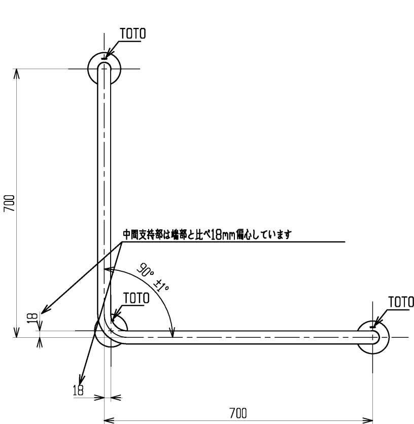
左壁設置の場合
