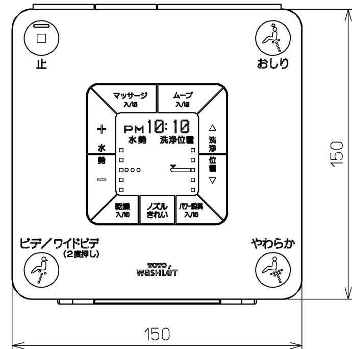
リモコン : 1個
