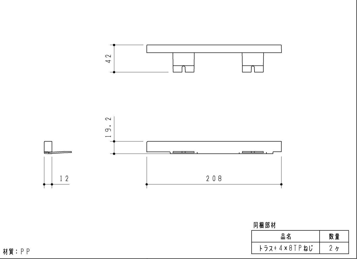
キャップセット(L)
