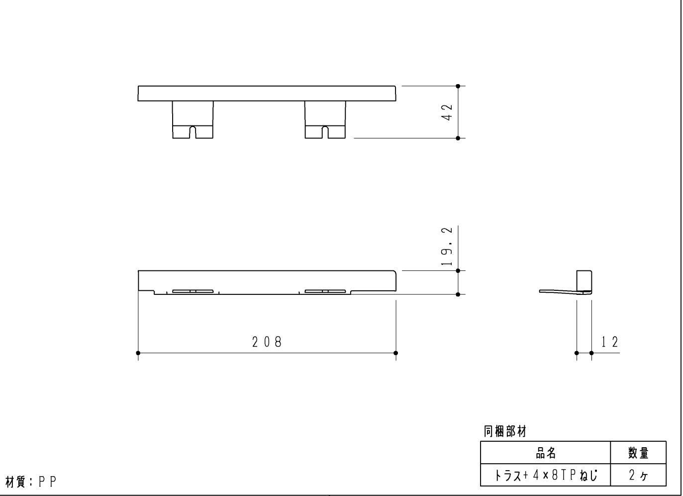
キャップセット(R)
