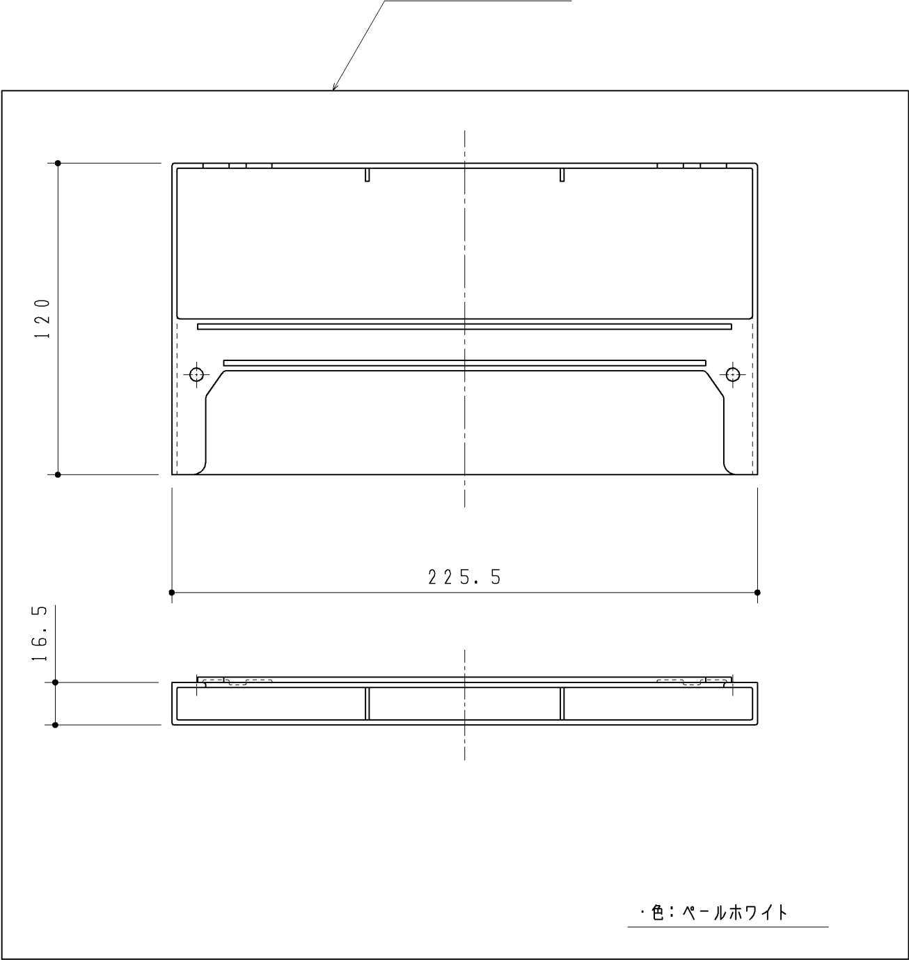
棚板キャップ(奥行大)
