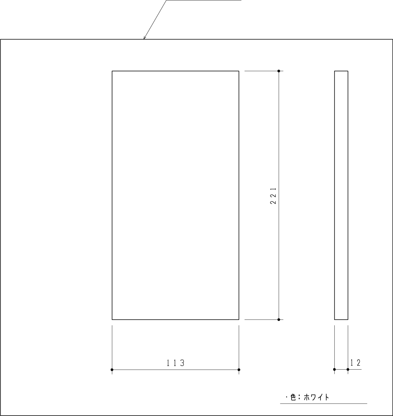
棚板(奥行大間口小)
