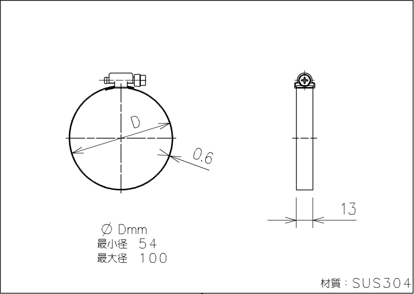
ホースクランプ
