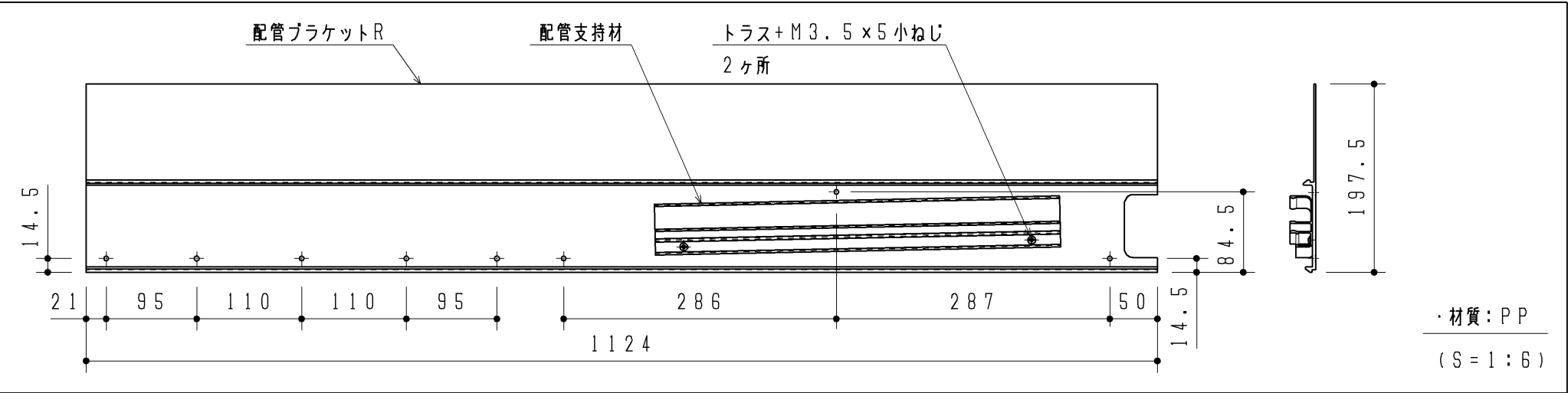
配管ブラケットセットR
