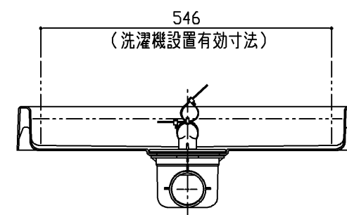
断面B-B
