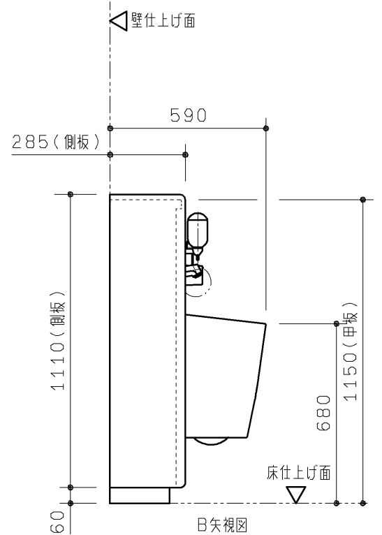
B矢視図
