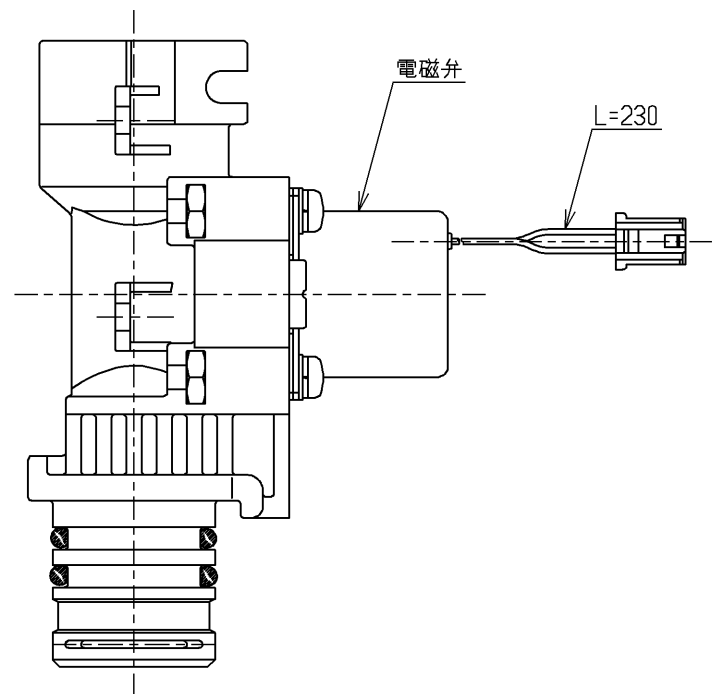
駆動部(水側)
