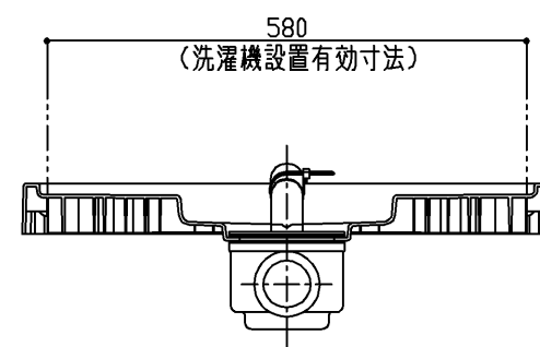
断面B-B
