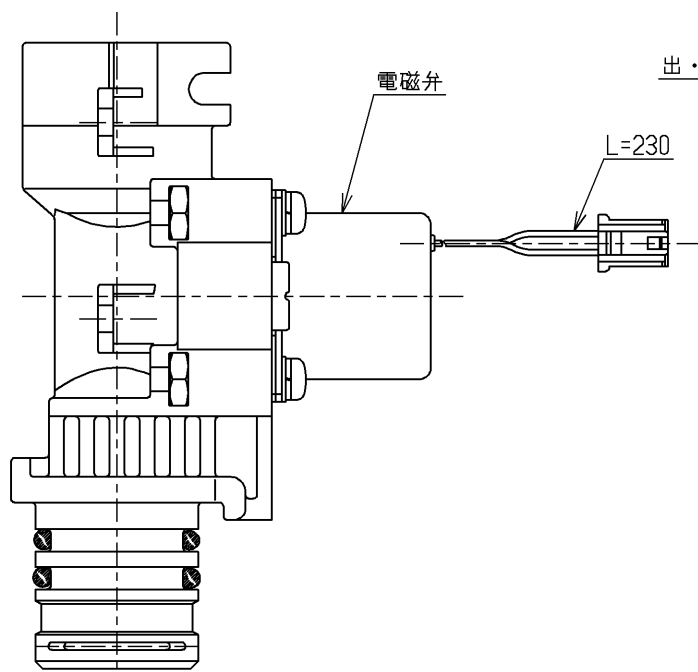
駆動部
