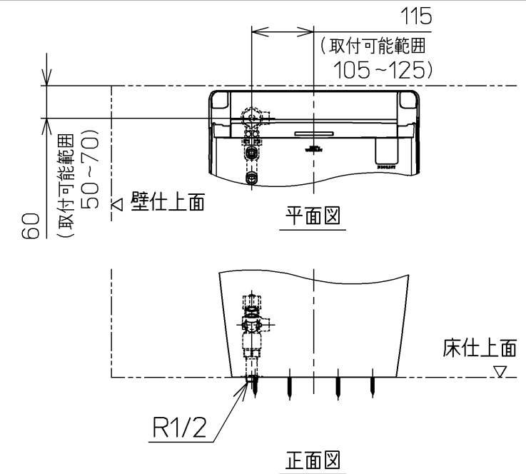
正面図 床給水仕様の場合
