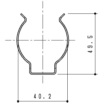
手洗器固定金具上
