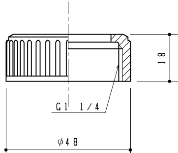
袋ナットG1（1/4）2ヶ
