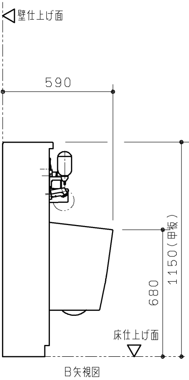
B矢視図
