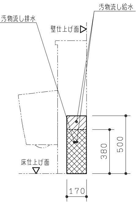
P 視図
