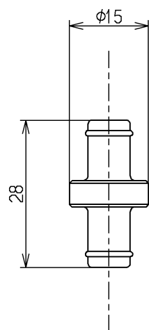
継手
