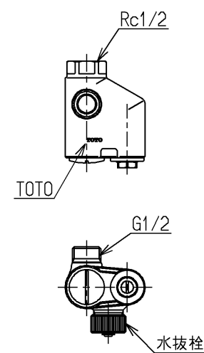
止水栓部(2ヶ)
