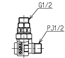
止水栓部 (2ヶ)
