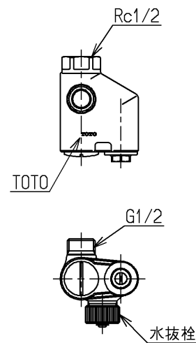
止水栓部(2ヶ)
