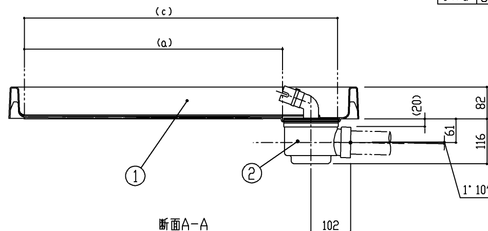
洗濯機設置有効寸法組合せ
